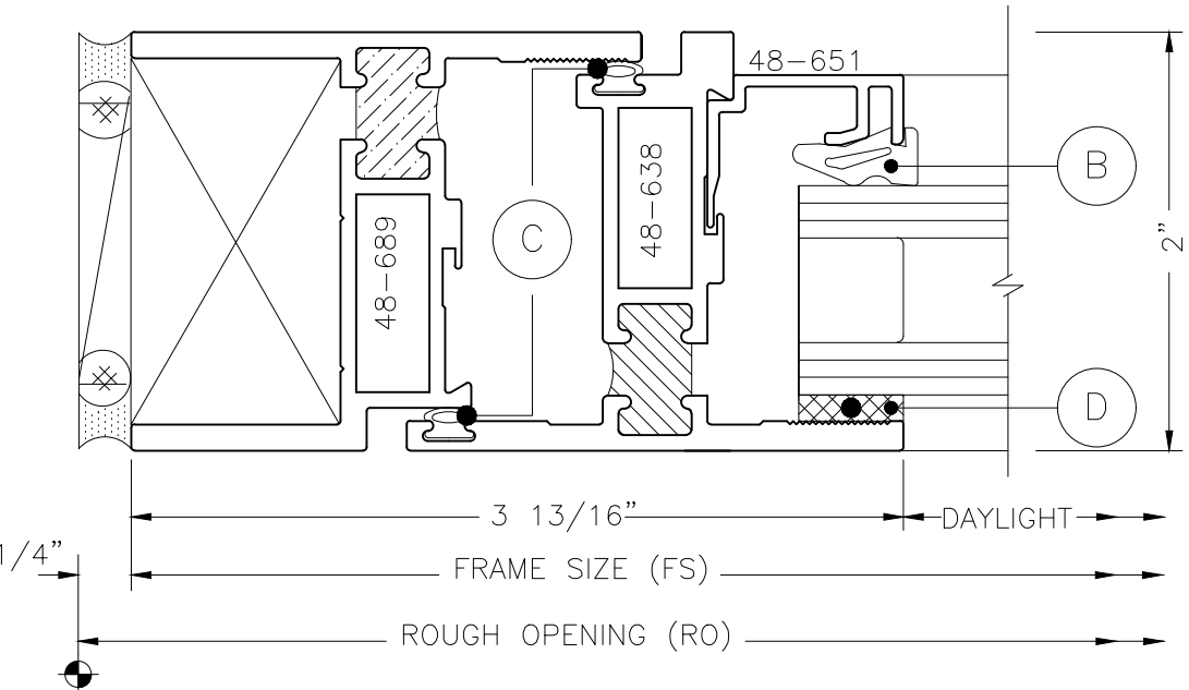
1" EXTENDED LEG JAMB
