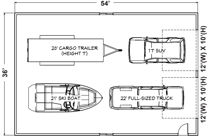
36'(W) x 54'(L) x 12' WALL
