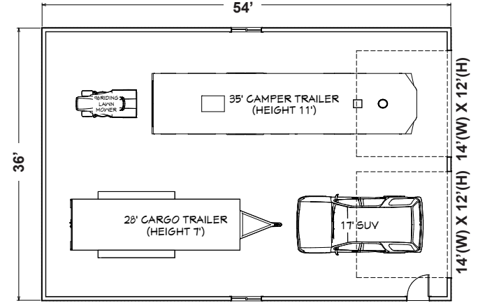
36'(W) x 54'(L) x 14' WALL
