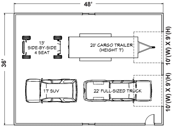
36'(W) x 48'(L) x 10' WALL
