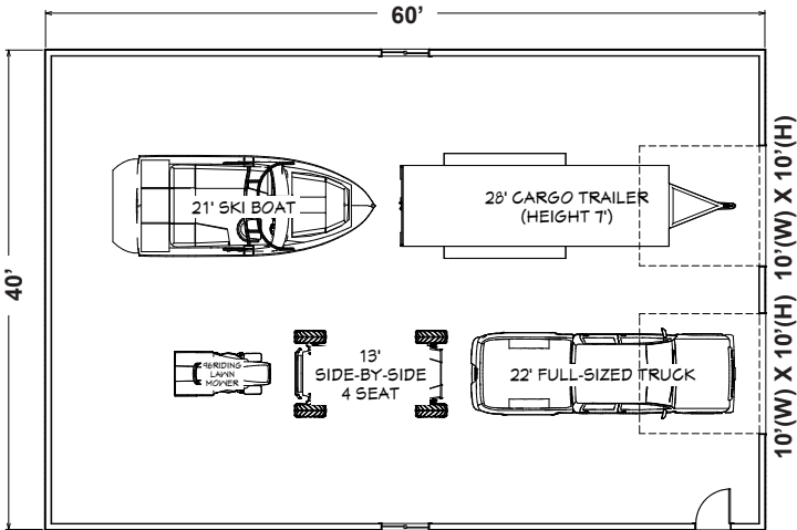
40'(W) x 60'(L) x 12' WALL
