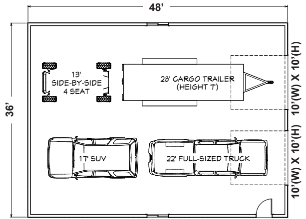
36'(W) x 48'(L) x 12' WALL
